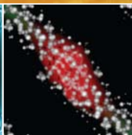
Molecules 001
